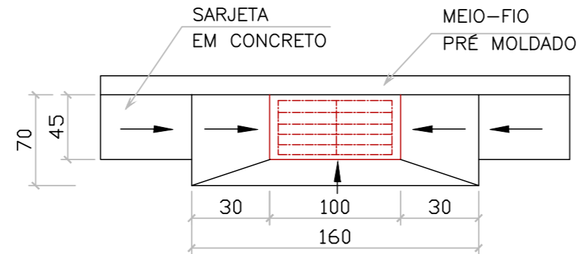
DEPRESSÃO DAS BOCAS-DE-LOBO-PLANTA sem escala
