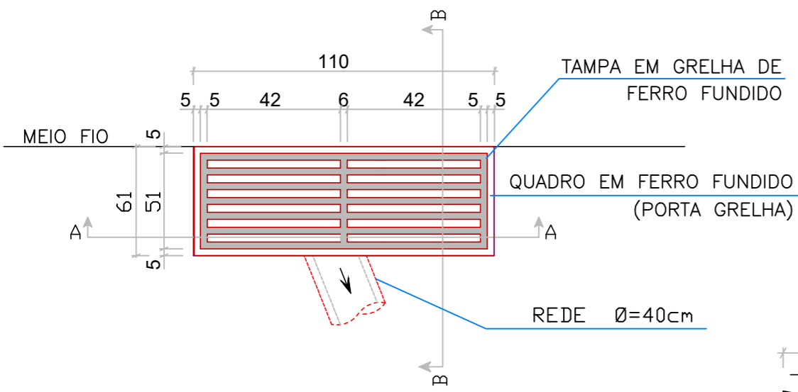
PLANTA BAIXA sem escala
