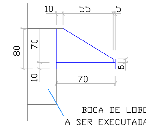
CORTE AA sem escala
